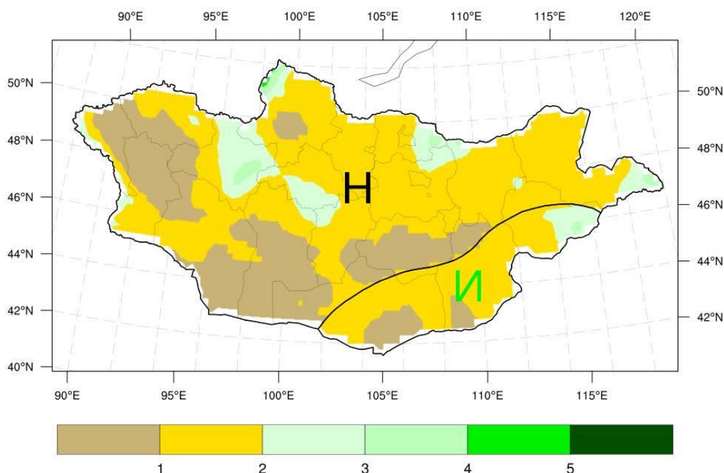
Зураг 2. 2025 оны 02-р сарын нийлбэр хур тунадасны урьдчилсан төлөв, мм
