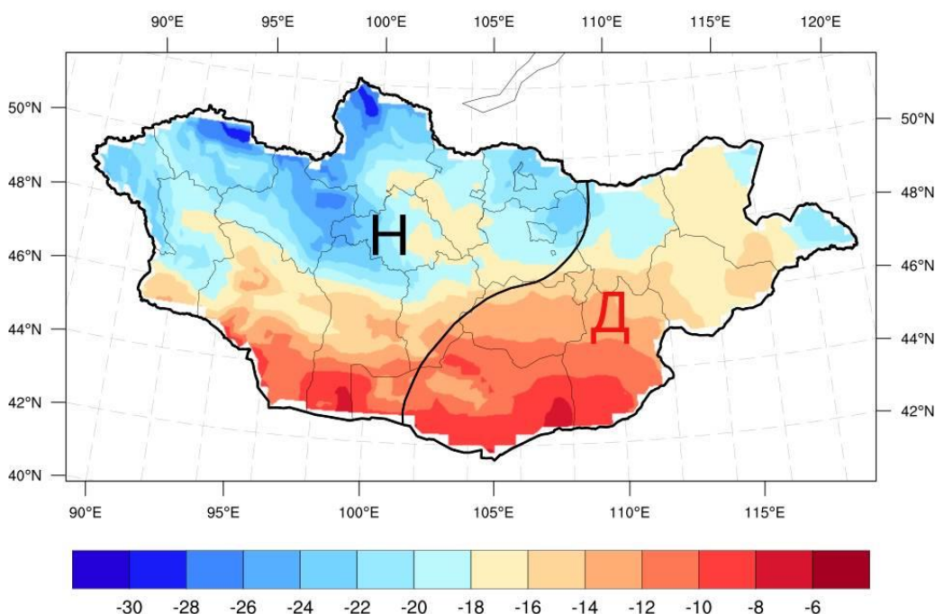
Зураг 1. 2025 оны 02-р сарын агаарын дундаж температурын урьдчилсан төлөв, C°
