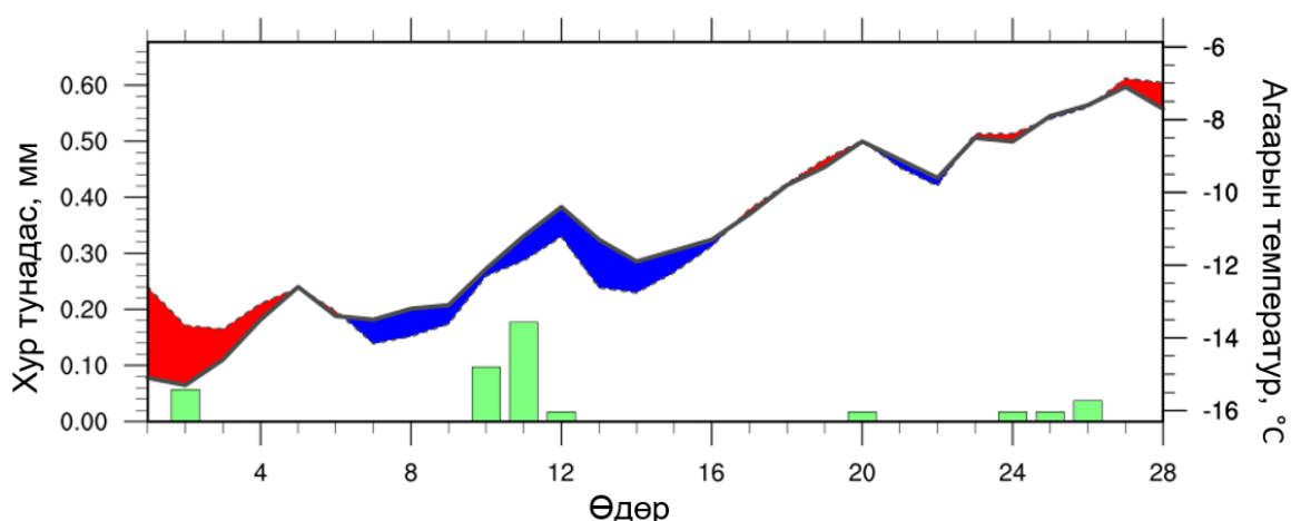
Зураг 3. Говийн аймгуудын нутгийн 2025 оны 02-р сарын температур, хур тунадасны явц
